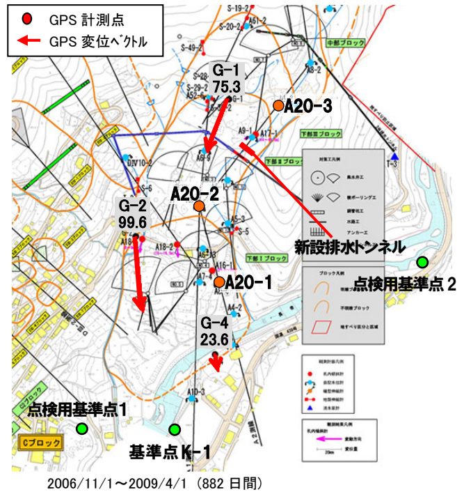
図-2 GPS 計測結果（平面変位ベクトル図）
