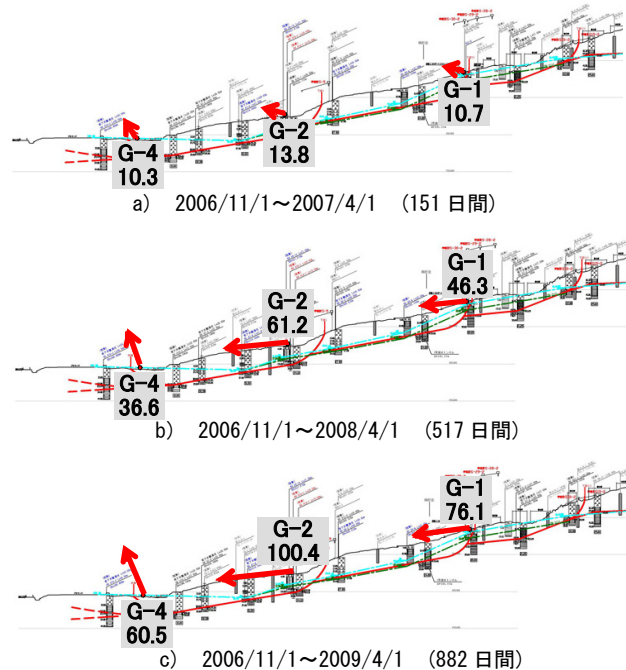
図-3 GPS 計測結果（断面変位ベクトル図）
